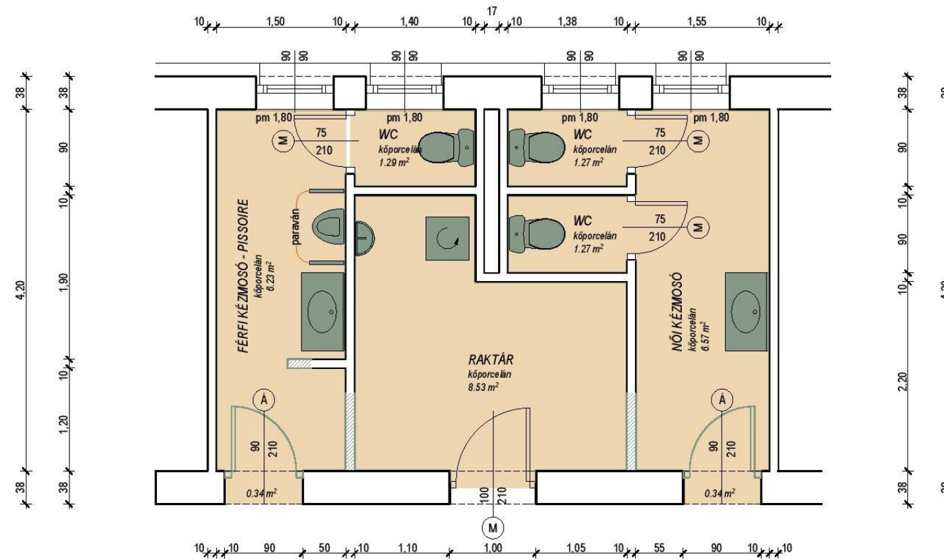
SZEMÉLYZETI MOSDÓ ALAPRAJZA
