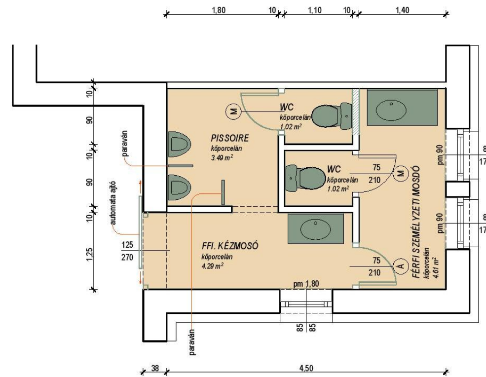
FÉRFI VIZESBLOKK ALAPRAJZA
