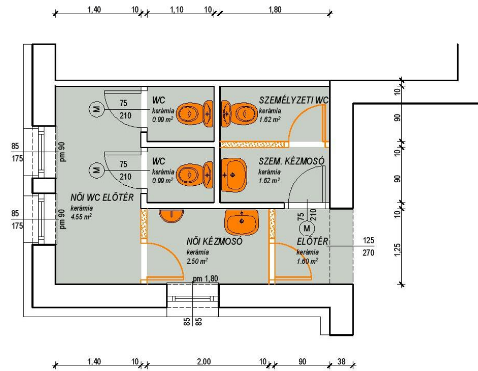
NŐI VIZESBLOKK ALAPRAJZA
